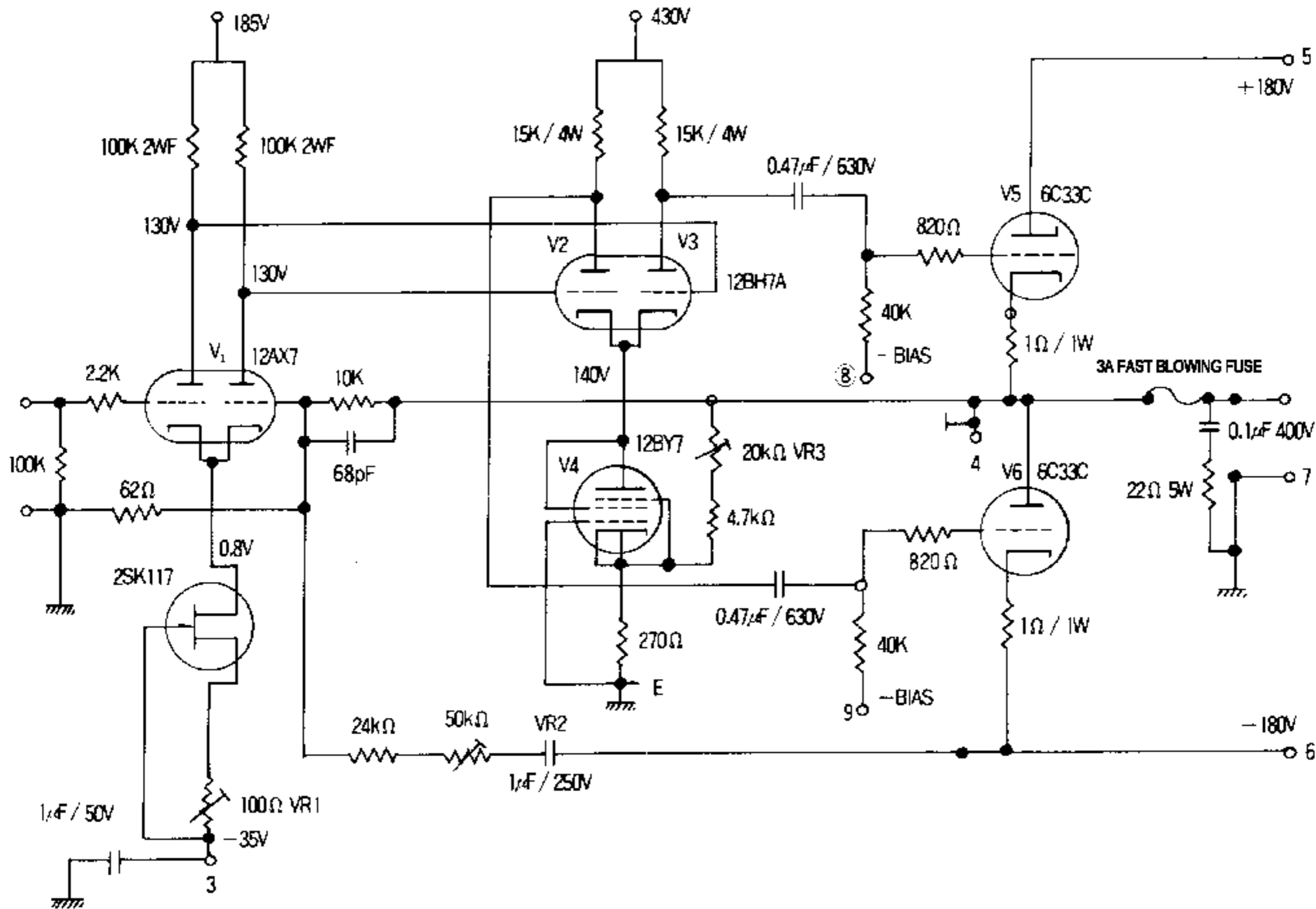
6C33CB-OTL MAIN
